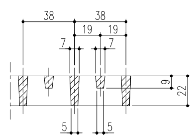
詳細図 S=1/2
