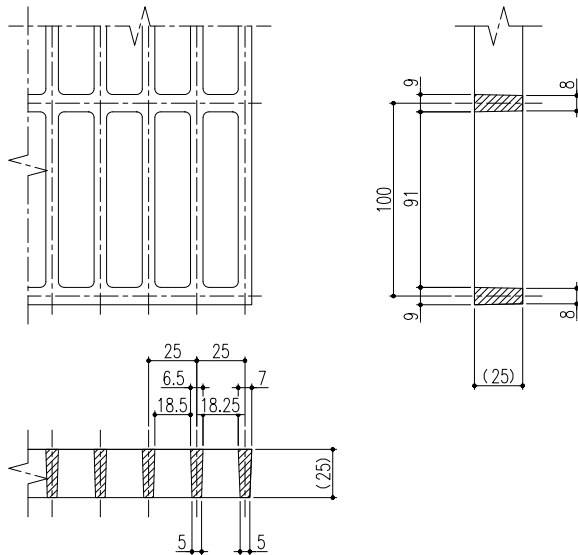
詳細図 S=1/2
