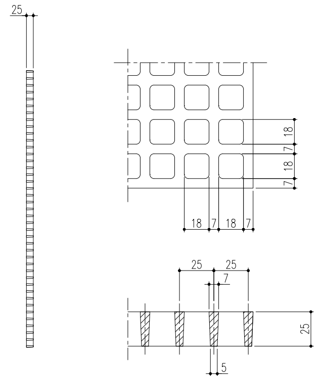
詳細図 S=1/2
